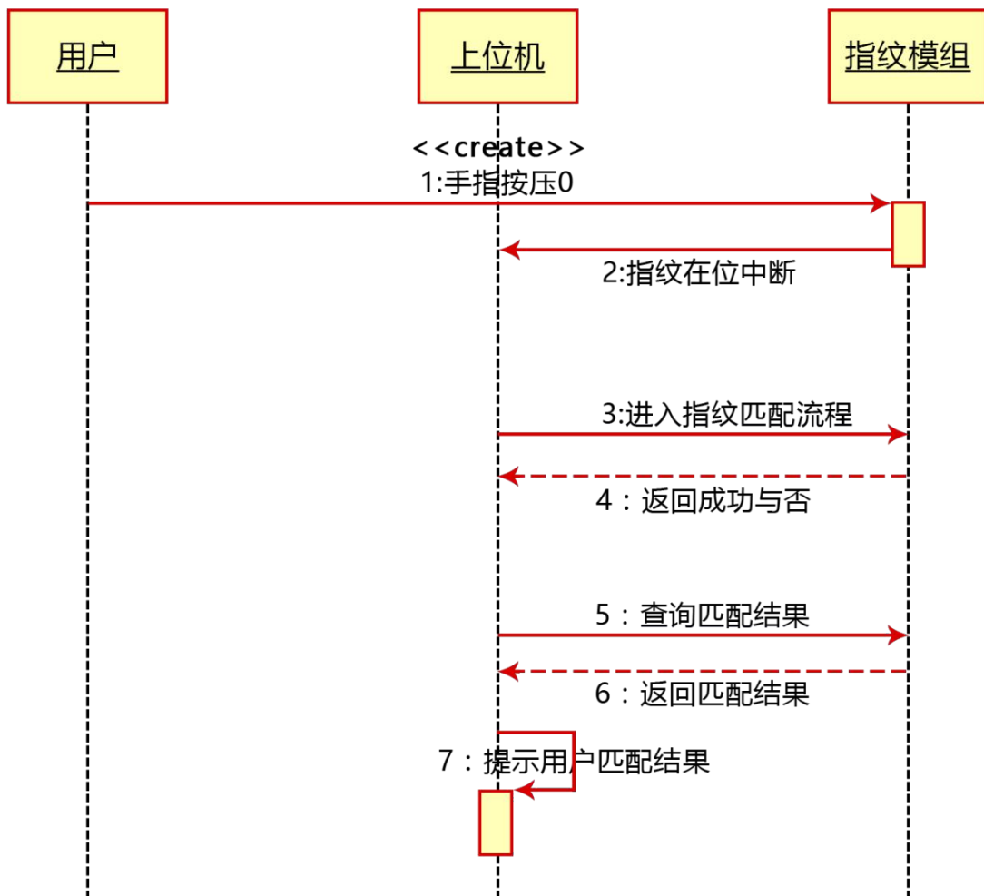
图 85 验证流程图
