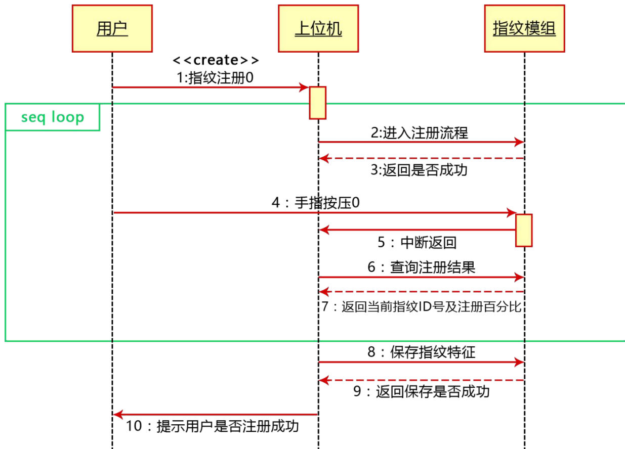
图 84 注册流程图
