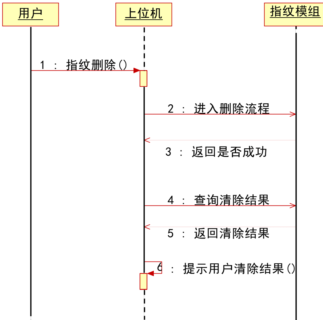
图 86 删除流程图
